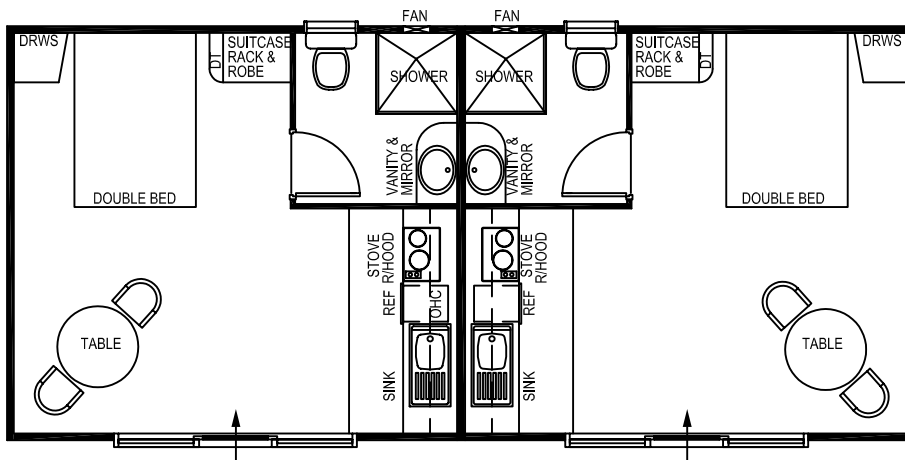
TUDOR 2 10.10x4.60 (31' x 15')
